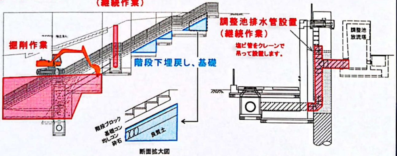
断面拡大図
