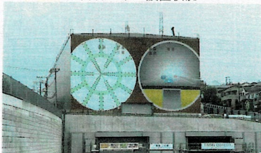
防音ハウス設置状況
