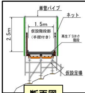
断面図
